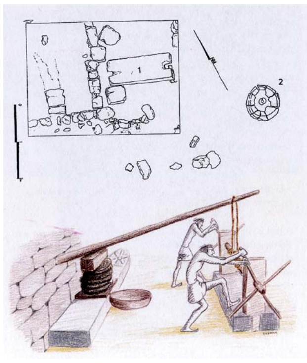
Fig. 7. Interpretació, que creiem més probable del torcularium per a l'elaboració de vi, amb elements aprofitats, en el paratge de la Fontjoana. (Dibuix de Julià Riu Serra).
